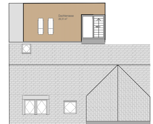
Grundriss Dachterrasse
