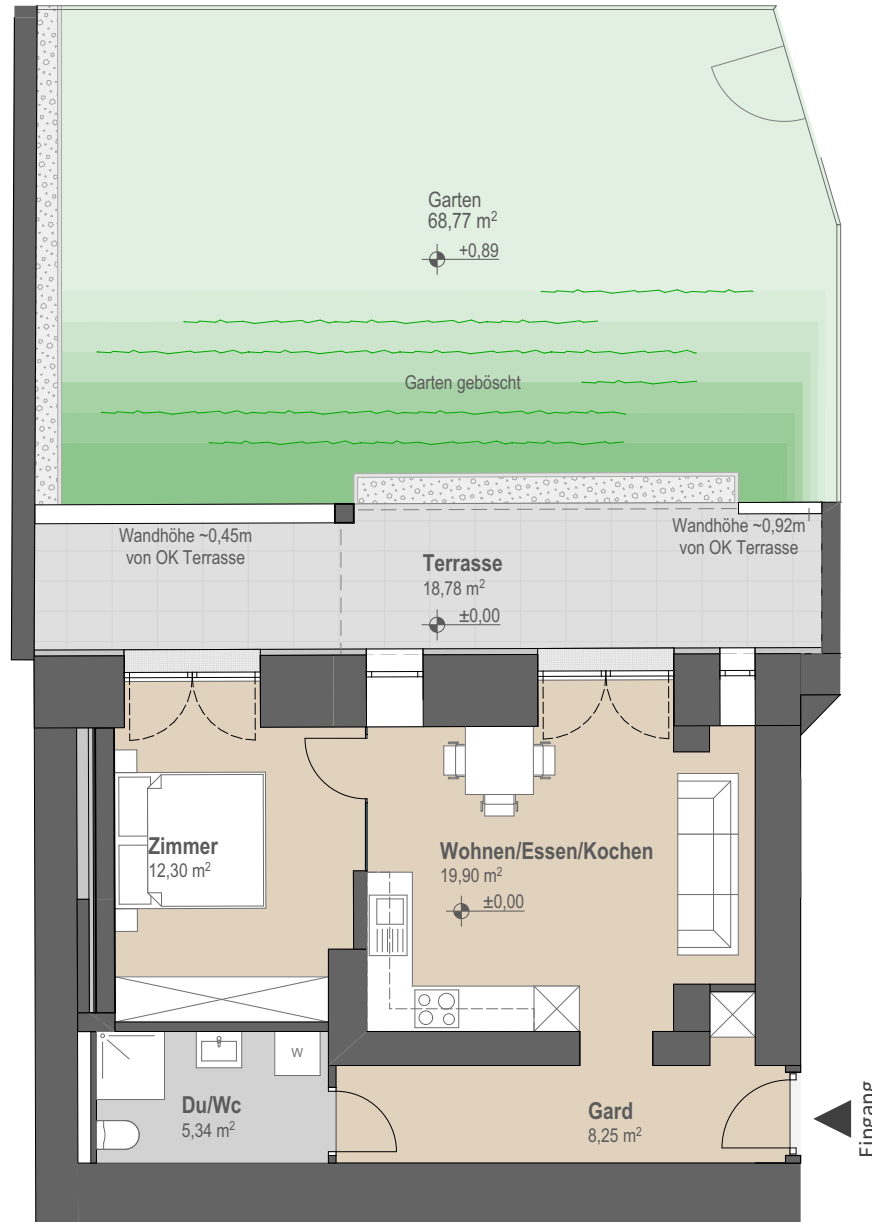
Grundriss Top G01 M 1:100
